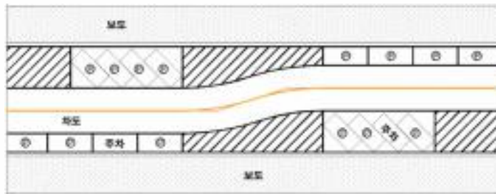
<그림 5-10> 지그재그 형태의 도로(평행주차, 45° 전진주차)
