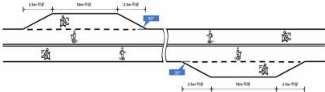
<그림 8-12> 양방향 양보차로형 추월차로
