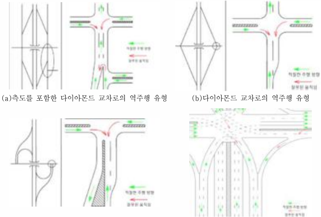
(c)부분 클로버형 역주행 유형
