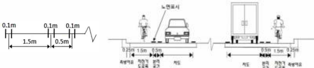
상세도
