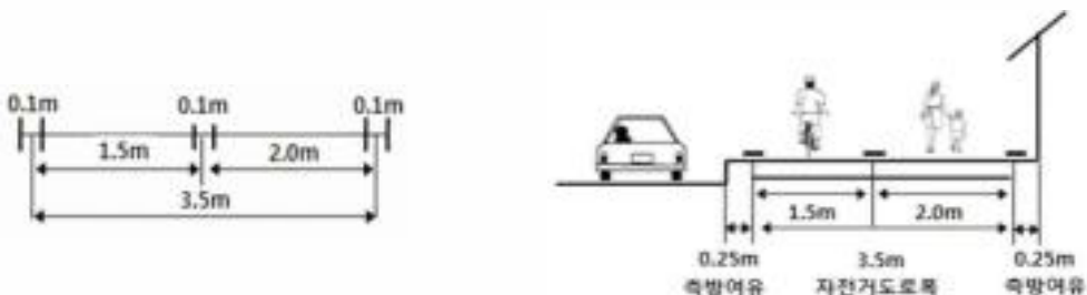
상세도
