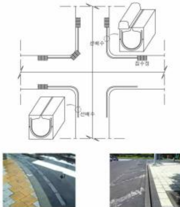
<그림 4-16> 교차로에서의 선배수 설치사례(예시)
