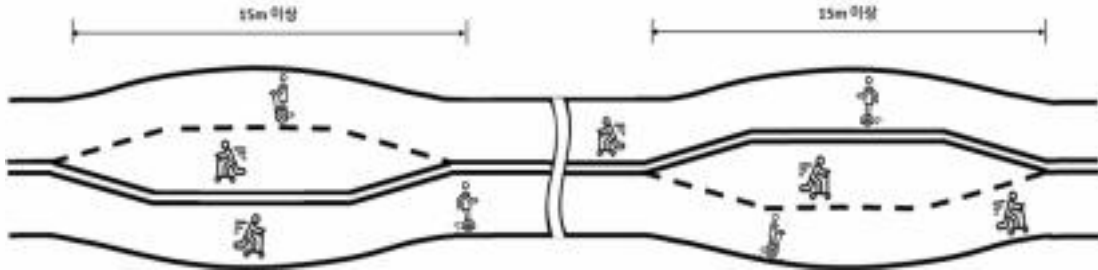
<그림 8-13> 2+1차로형 추월차로
