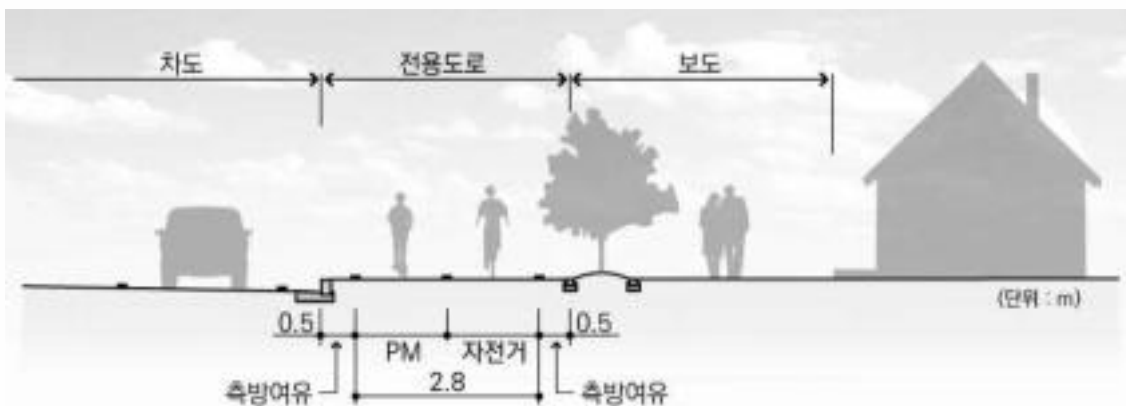
<그림 8-2> PM을 고려한 자전거 전용도로 횡단 예시(일방향)
