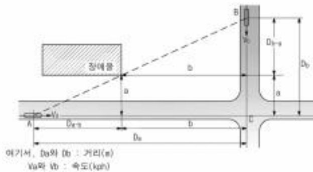
<그림 5-20> 평면교차로 시거 삼각형
