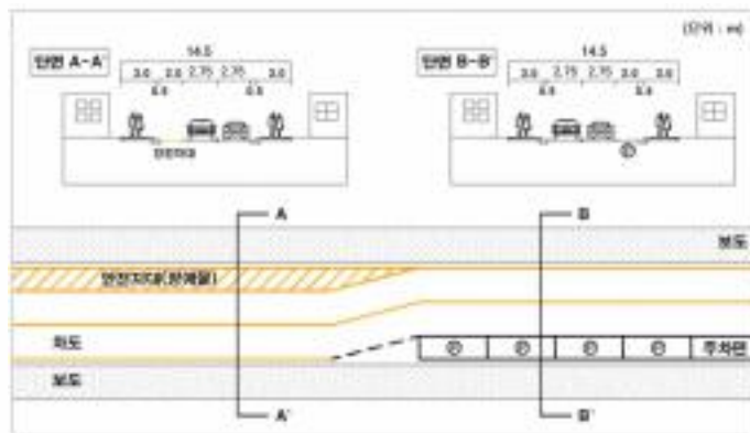
<그림 5-11> 지그재그 형태의 도로(평행주차)
