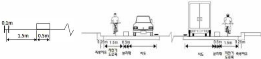
상세도
