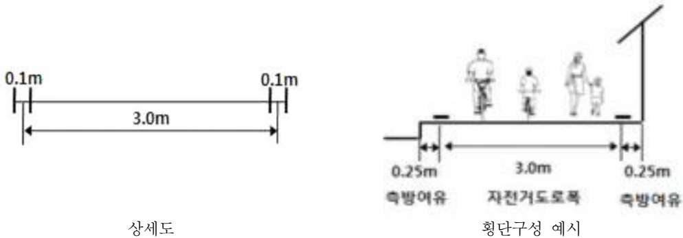
<그림 3-8> 자전거도로와 보도 비분리 설치 시 횡단구성(예시)
