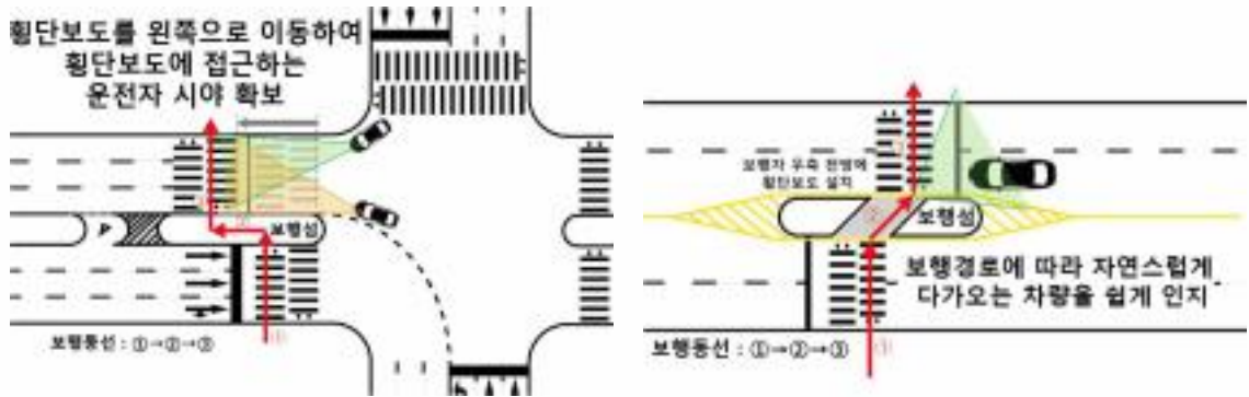
(a) 교차로에서 먼 쪽으로 횡단보도 설치(교차로) (b) 보행자 우측 전방 횡단보도 설치(단일로)
