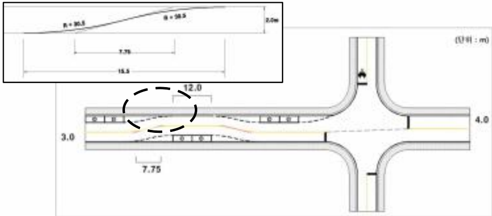
<그림 5-15> 지그재그 형태의 도로(교차로 진입부 주차면 설계)
