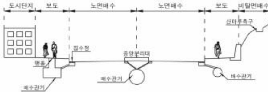
<그림 4-15> 도시지역도로 배수시설(예시)
