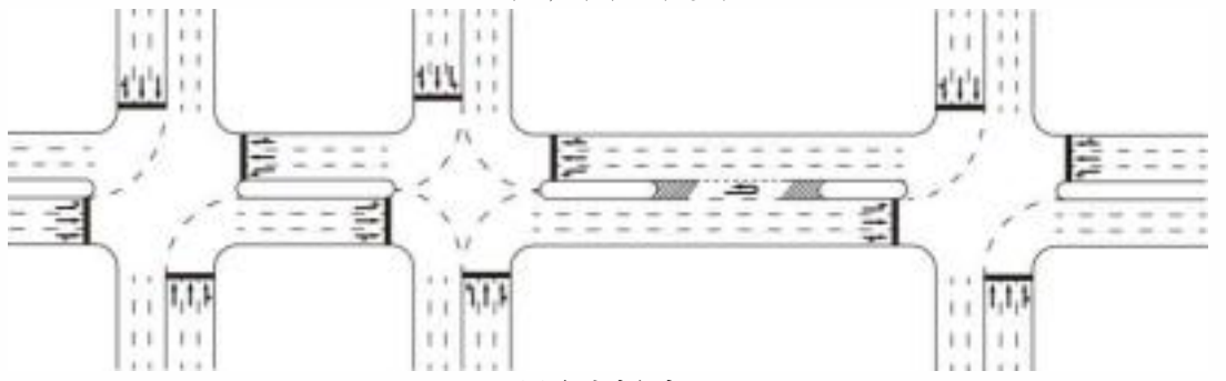
(b)유턴전용차로
