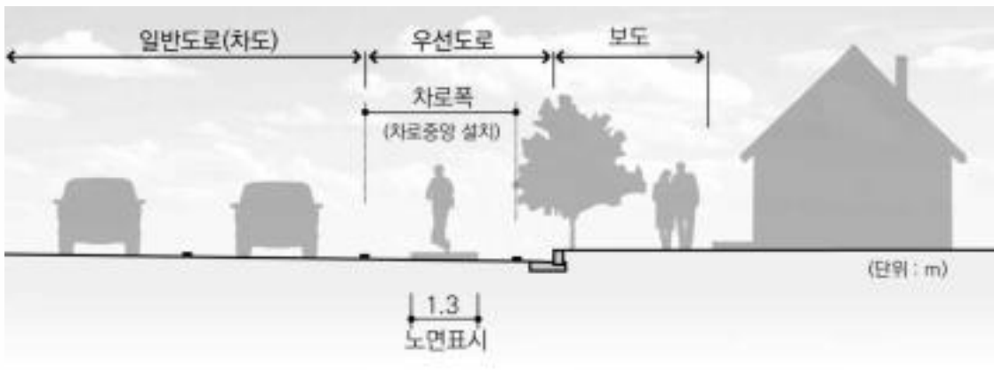
<그림 8-6> PM을 고려한 자전거 우선도로 횡단 예시
