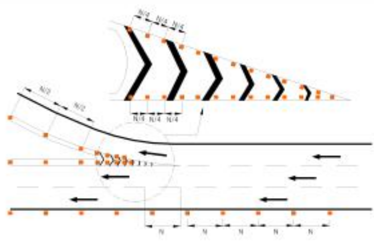
(a) 고속도로 진·출입연결로에서의 표지병 설치방법
