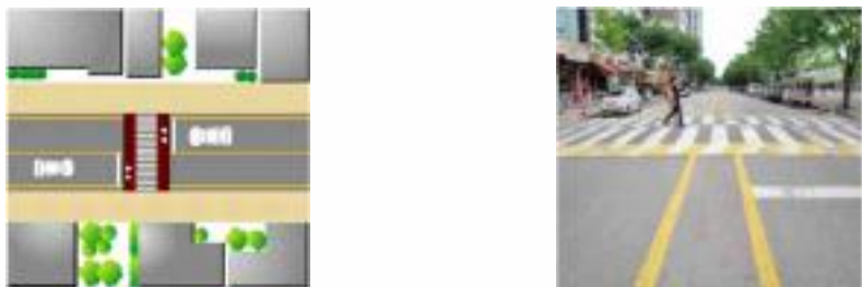
<그림 4-9> 고원식 횡단보도 설치 예시
