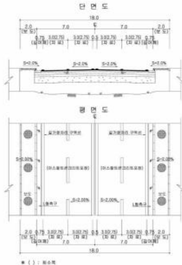
<그림 3-24> 설계속도 시속 30킬로미터일 때 도로 폭 예시도 (B=18.0m, 왕복 4차로)
