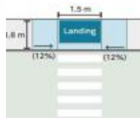
보도전체 턱낮춤
