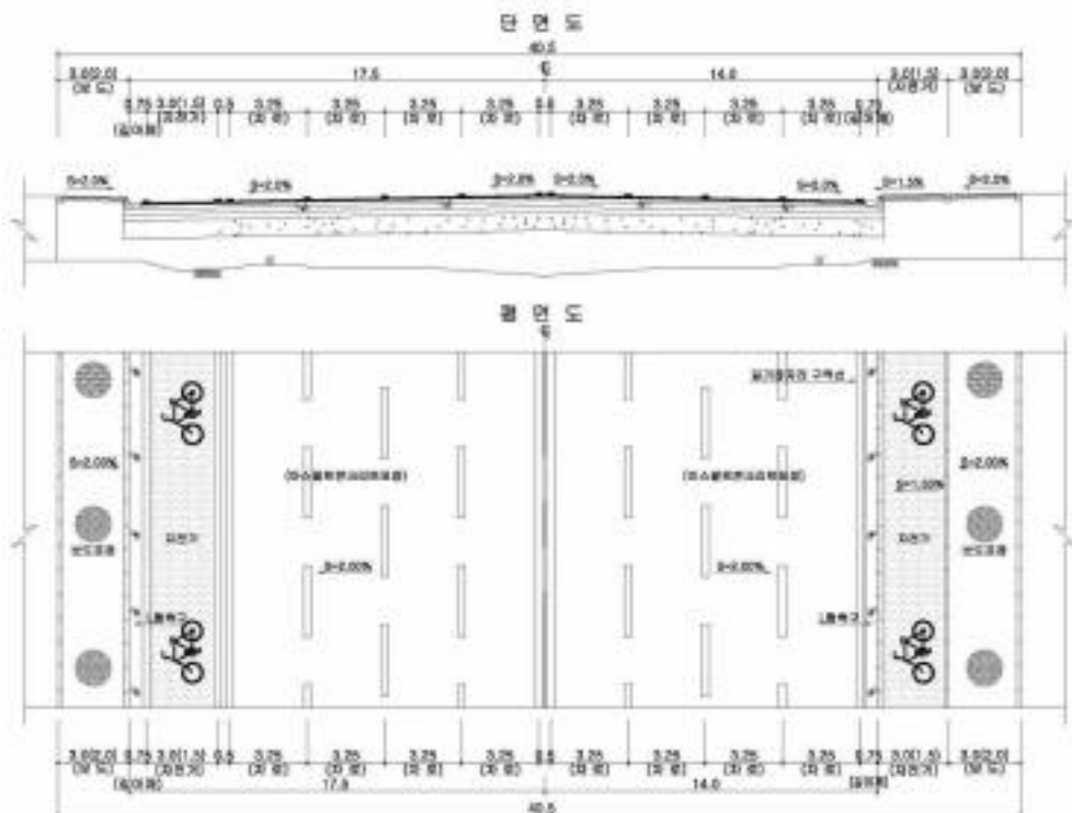
<그림 3-18> 설계속도 시속 50킬로미터일 때 자전거도로 설치 예시도(B=40.5m, 왕복 8차로)
